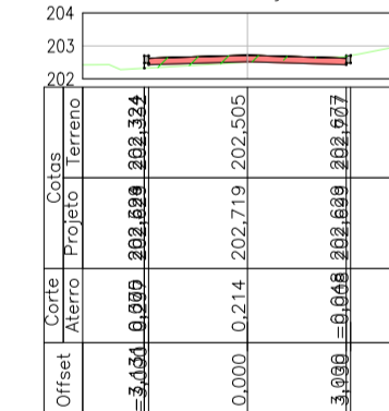
Alinhamento - Rua Projetada C - 9+0.00
