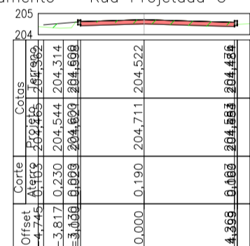
Alinhamento - Rua Projetada C - 2+20.00
