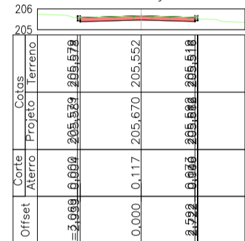
Alinhamento - Rua Projetada B - 2+0.00
