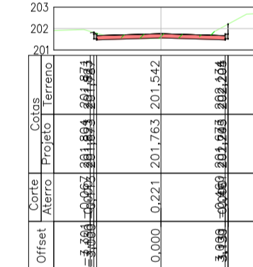
Alinhamento - Rua Projetada C - 10+0.00
