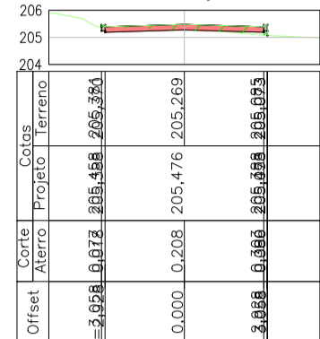
Alinhamento - Rua Projetada B - 3+0.00
