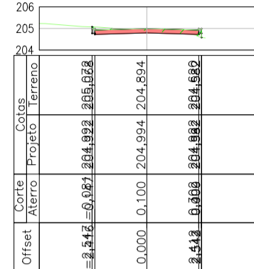
Alinhamento - Rua Projetada B - 6+0.00
