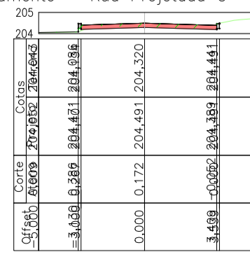
Alinhamento - Rua Projetada C - 3+20.00
