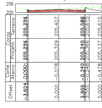
Alinhamento - Rua Projetada C - 0+20.00
