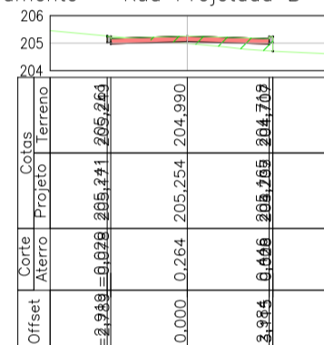
Alinhamento - Rua Projetada B - 4+0.00
