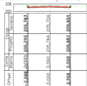
Alinhamento - Rua Projetada B - 1+0.00
