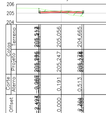
Alinhamento - Rua Projetada B - 4+20.00
