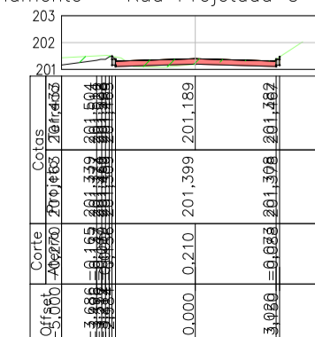
Alinhamento - Rua Projetada C - 11+0.00
