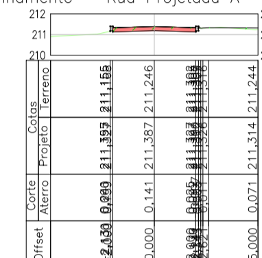
Alinhamento - Rua Projetada A - 4+0.00
