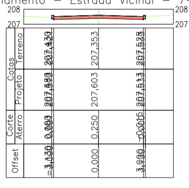
Alinhamento - Estrada Vicinal - 7+0.00
