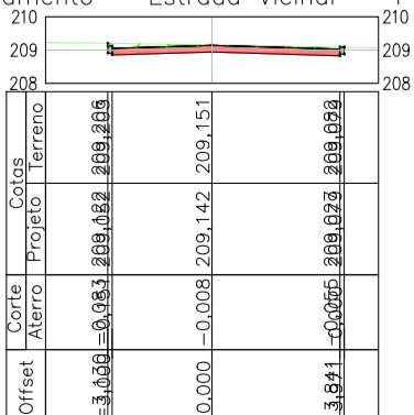
Alinhamento - Estrada Vicinal - 1+0.00
