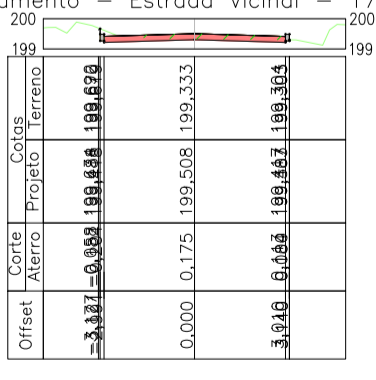
Alinhamento - Estrada Vicinal - 17+0.00
