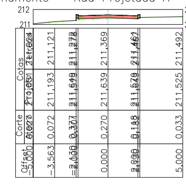
Alinhamento - Rua Projetada A - 3+0.00
