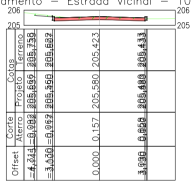
Alinhamento - Estrada Vicinal - 10+0.00
