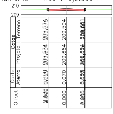
Alinhamento - Rua Projetada A - 14+0.00
