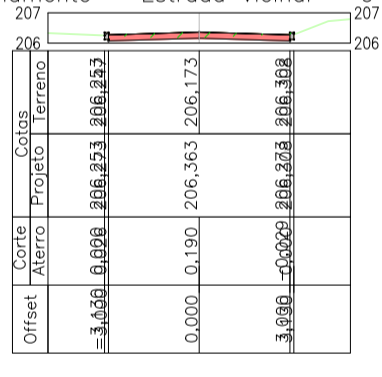
Alinhamento - Estrada Vicinal - 9+0.00
