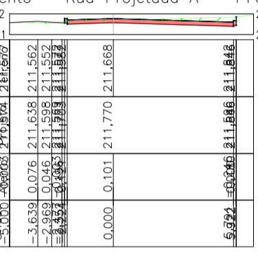
Alinhamento - Rua Projetada A - 1+0.00
