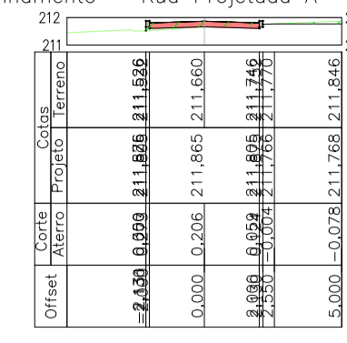
Alinhamento - Rua Projetada A - 6+0.00
