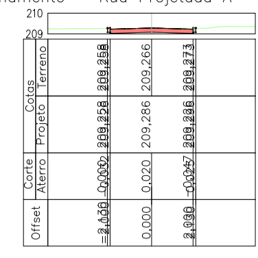
Alinhamento - Rua Projetada A - 15+0.00
