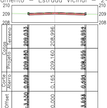
Alinhamento - Estrada Vicinal - 2+0.00
