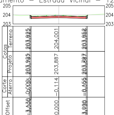
Alinhamento - Estrada Vicinal - 12+0.00
