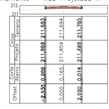
Alinhamento - Rua Projetada A - 8+0.00
