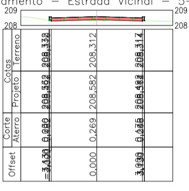
Alinhamento - Estrada Vicinal - 5+0.00
