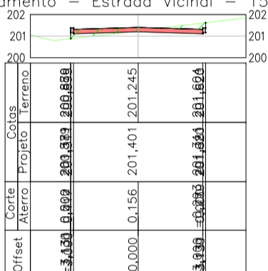
Alinhamento - Estrada Vicinal - 15+0.00
