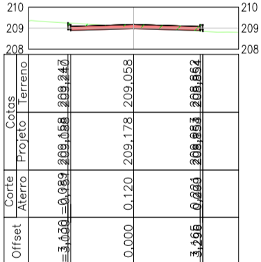
Alinhamento - Estrada Vicinal - 3+0.00
