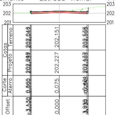
Alinhamento - Estrada Vicinal - 14+0.00
