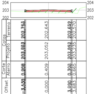
Alinhamento - Estrada Vicinal - 13+0.00
