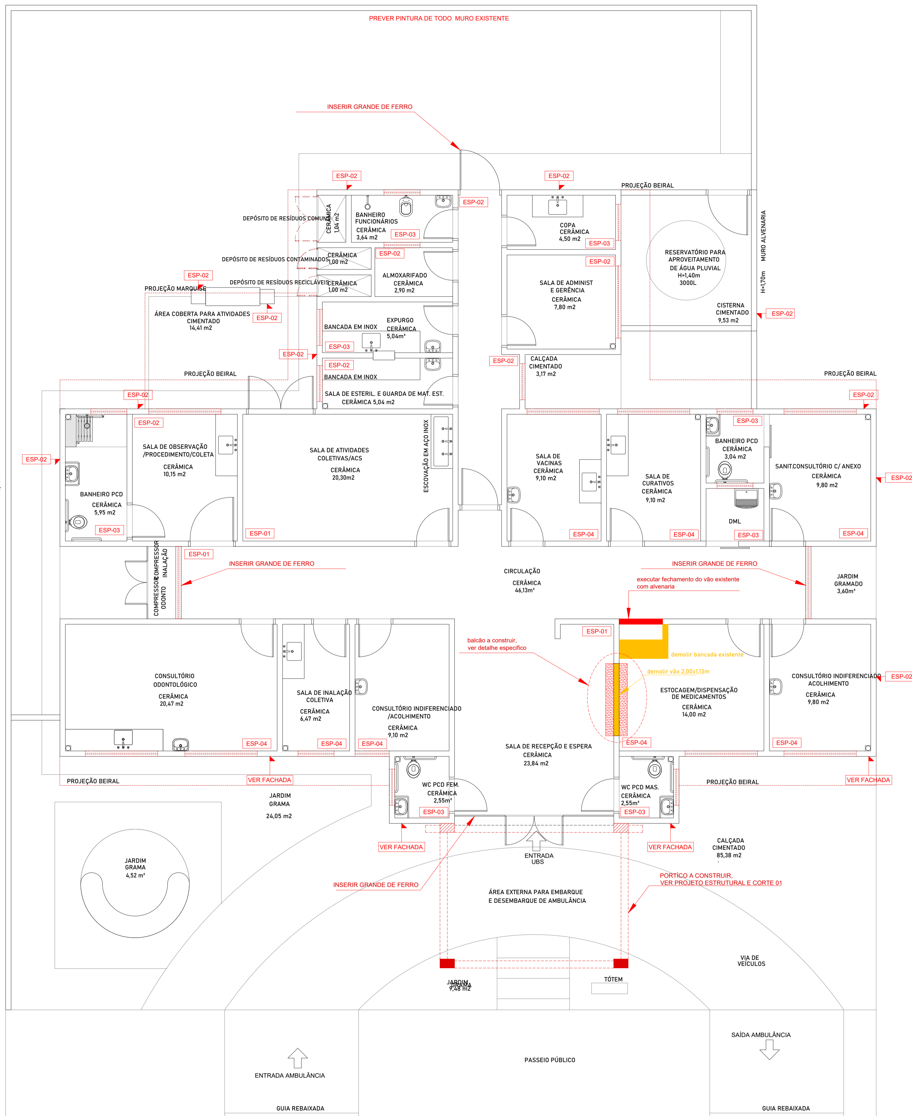
PLANTA BAIXA INTERVENÇÕES ESC 1/75
